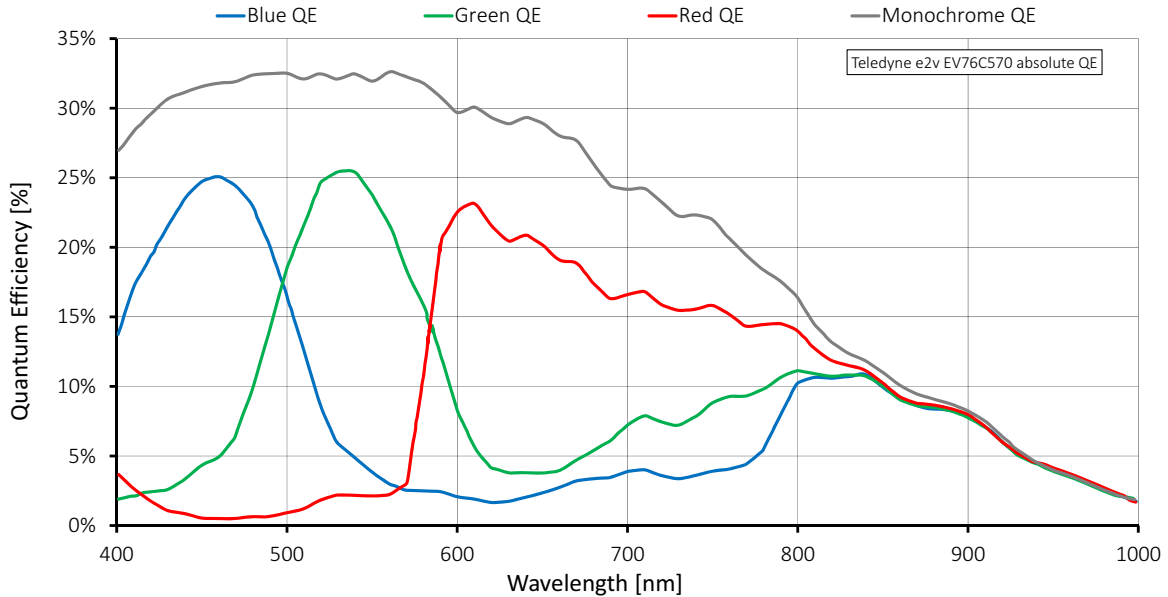
Figure 21: Mako G-192 (Teledyne e2v EV76C570) absolute QE
